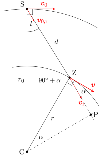
Slika 3. Zvezda Z z galaktično širino l , ki kroži okoli središča Galaksije C , se glede na Sonce S giblje z radialno hitrostjo v'_r , ki je razlika projekcij v_r in v_{0,r} hitrosti kroženja zvezde in Sonca na opazovalčevo smer pogleda.
