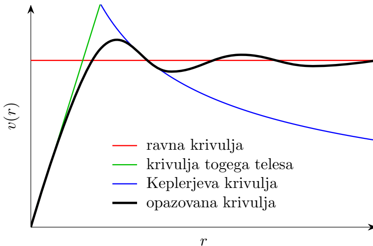
Slika 7. Rotacijska krivulja. Prikazana je krožna hitrost v(r) kot funkcija galaktičnega radija r . V notranjosti Galaksije (do približno 2–3 kpc) hitrost hitro narašča, kar ustreza rotaciji togega telesa. V zunanjem disku (od približno 3 kpc naprej) pa je krivulja skoraj ravna, kar nakazuje na prisotnost temne snovi. Skica: Žan Arsov.
