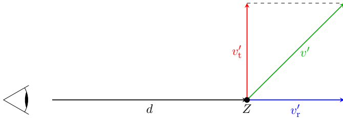
Slika 2. Relativno hitrost v' zvezde glede na opazovalca lahko zapišemo kot vektorsko vsoto radialne komponente v'_r , ki jo izračunamo na podlagi meritev Dopplerjevega premika spektralnih črt, in tangentno komponento v'_t , ki jo izračunamo na podlagi meritev lastnega gibanja \mu .
