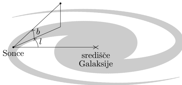
Slika 1. V galaktičnem koordinatnem sistemu položaj zvezde opišemo z galaktično dolžino l in galaktično širino b . Skica: Žan Arsov.
