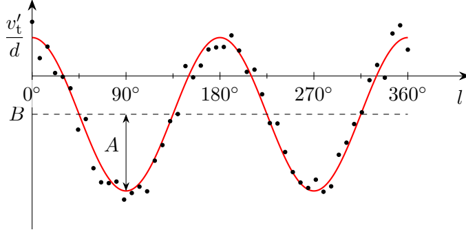
Slika 5. Relativna tangentsna hitrost v'_t zvezd v Sončevi okolici v odvisnosti od galaktične dolžine l . Na grafu je kosinusna krivulja z amplitudo, določeno z Oortovo konstanto A , ki je glede na vodoravnico zamaknjena za vrednost Oortove konstante B . Podatki so simulirani in služijo zgolj za grafično ponazoritev pričakovane odvisnosti. Skica: Žan Arsov.
