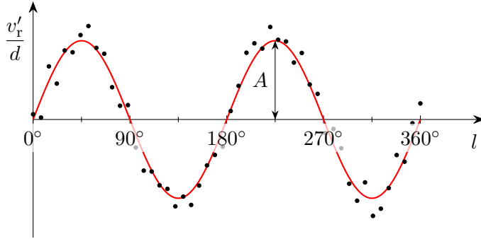
Slika 4. Relativna radialna hitrost v'_r zvezd v Sončevi okolici v odvisnosti od galaktične dolžine l . Amplituda sinusne krivulje ponazarja Oortovo konstanto A . Podatki so simulirani in služijo zgolj za grafično ponazoritev pričakovane odvisnosti. Skica: Žan Arsov.
